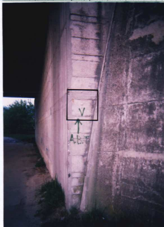
FOTO 2 : CAPOSALDO VERTICALE
